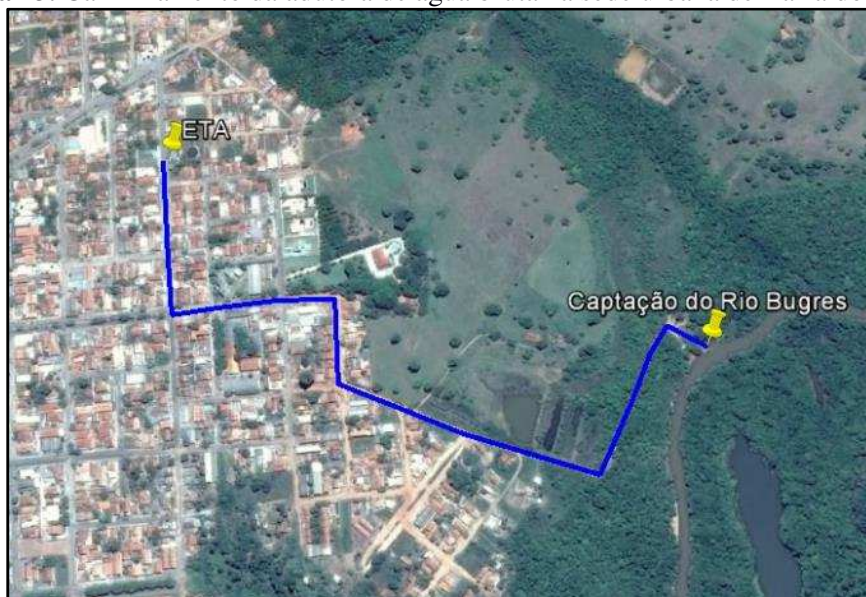
Figura 13. Caminhamento da adutora de água bruta na sede urbana de Barra do Bugres
