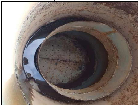
Figura 115. Filtro da ETA de Assari inoperante devido a problemas estruturais
