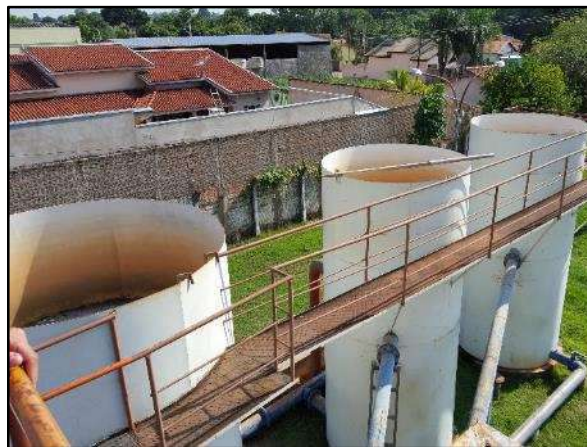
Figura 30. Filtros de múltiplas camadas com fluxo descendentes da ETA metálica
