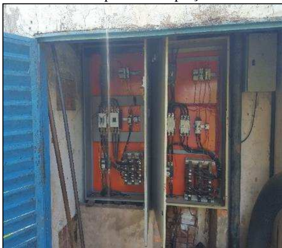
Figura 16. Quadro de comando protegido de intempéries da captação
