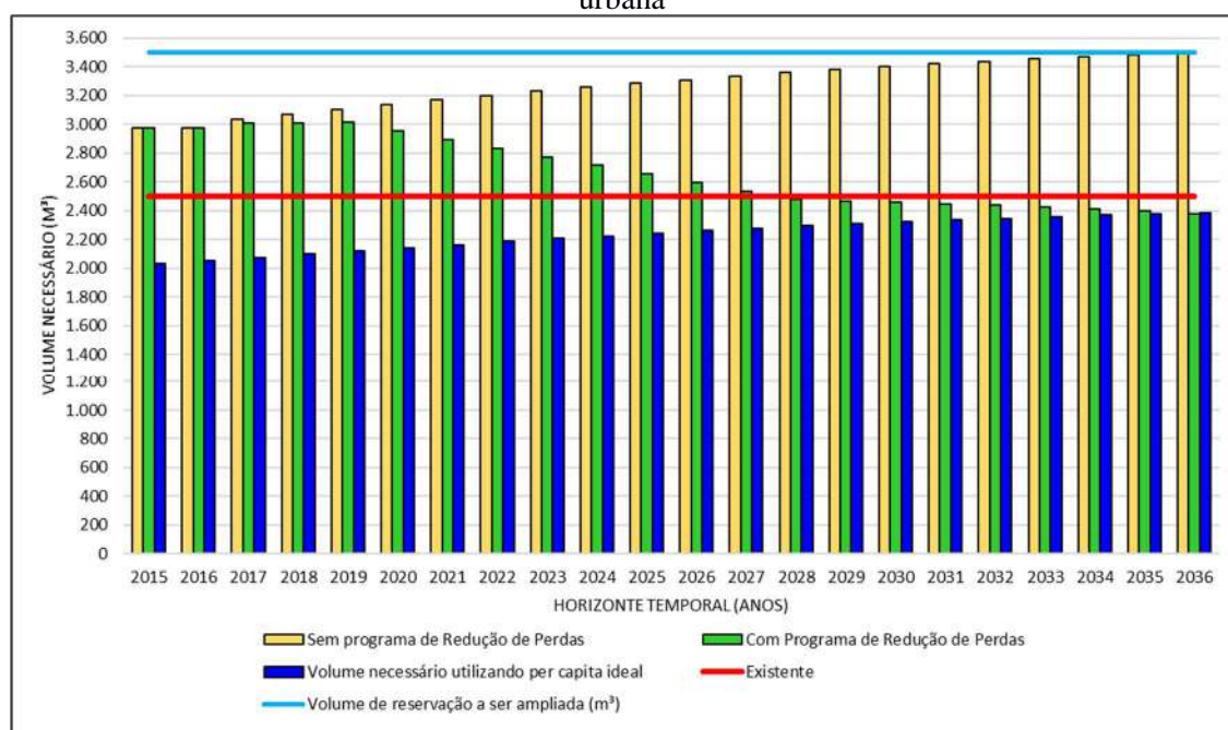
Figura 152. Gráfico do volume de reservação necessária para atendimento da demanda da sede urbana
