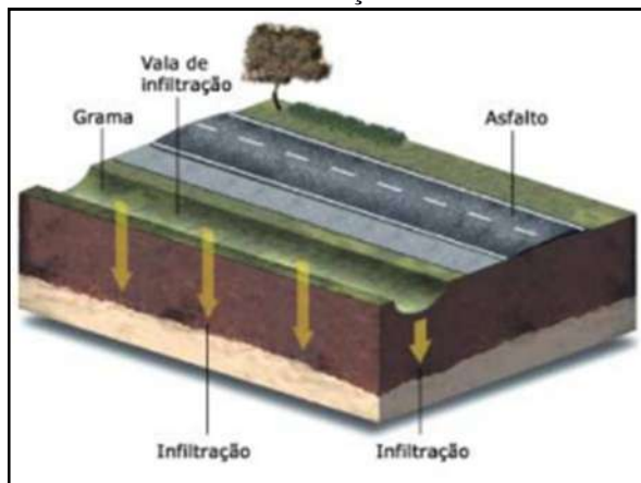
Figura 179. Esquema de funcionamento de vala de infiltração
