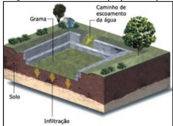
Figura 181. Reservatório em parque municipal
